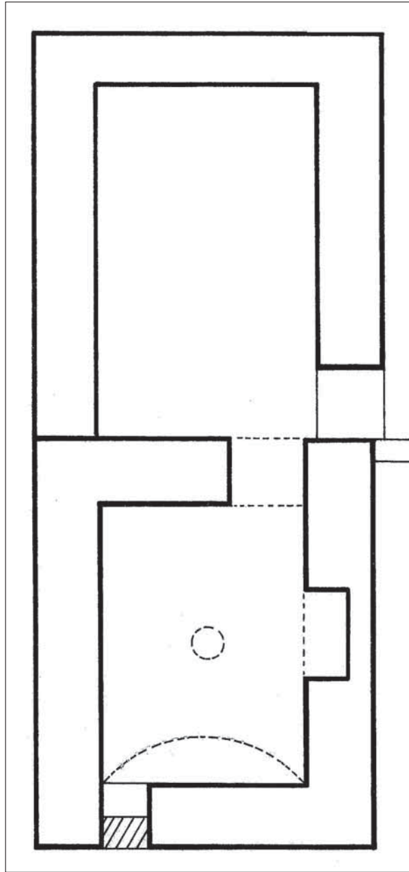
Lev. 157 ŞARKIKARAAĞAÇ ILICASI RÖLÖVE PLANI RLV: B. AÇIKYILDIZ, H. EYİER, E. GÜREL, N. ŞAMAN ÇZN: Y. KILIÇ
