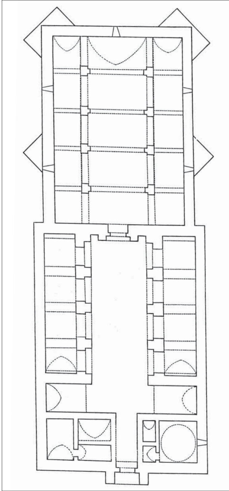
LEV. 170 GELENDOST ERTOKUŞ HAN RESTİTÜSYONU (K. ERDMANN 1961)
