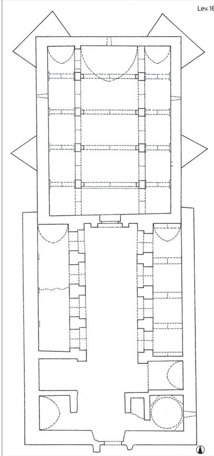
LEV. 169 GELENDOST ERTOKUŞ HAN RÖLÖVE PLANI RLV: B. AÇIKYILDIZ, V. HASBAY, N. ŞAMAN, E. TAŞDELEN, T. YAZAR ÇZN: T. YAZAR
